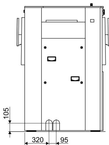
Näkymä vasemmalta
